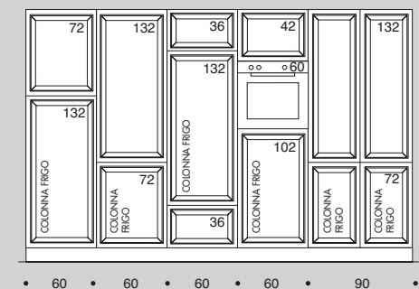
COLONNE FRIGO REFRIGERATOR TALL UNITS ARMOIRES POUR REFRIGERATEUR H 204cm
