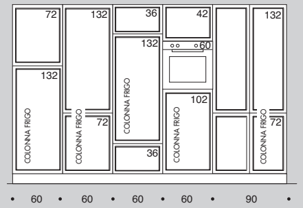
COLONNE FRIGO REFRIGERATOR TALL UNITS ARMOIRES POUR REFRIGERATEUR H 204cm
