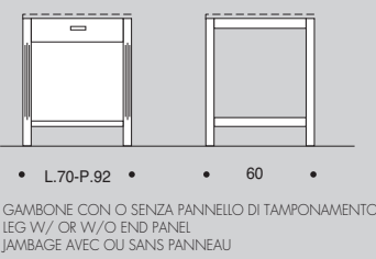
BASI A GIORNO OPEN BASE ELEMENTS BAS OUVERTS
