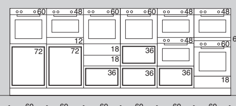
COLONNE FORNO OVEN TALL UNITS ARMOIRES POUR FOUR H 132cm
