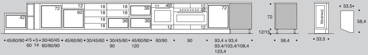
BASI A GIORNO OPEN BASE ÉLÉMENTS BAS OUVERTS
