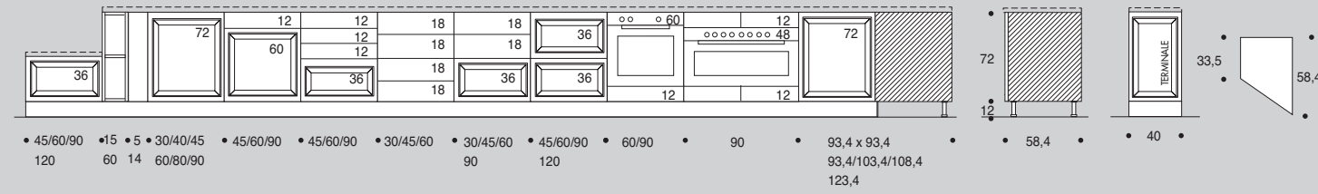
BASI ATTEZZATE EQUIPPED BASES BASES EQUIPES
