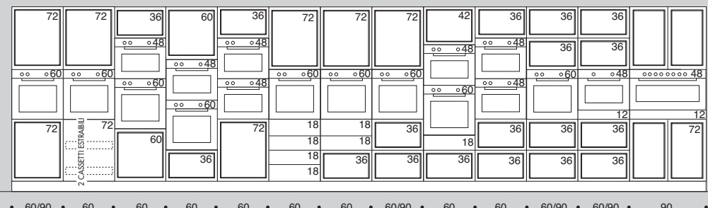
COLONNE FORNO OVEN TALL UNITS ARMOIRES POUR FOUR H 204cm
