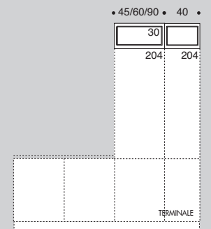
SOPRAPENSILE E SOPRACOLONNE SUSPENDED WALL UNIT AND TALL UNITS ELEMENTS SUR MEUBLES HAUTS ET SUR ARMOIRES
