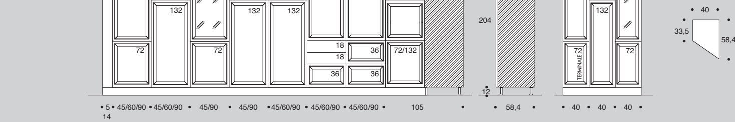
COLONNE ATTEZZATE EQUIPPED TALL UNITS ARMOIRES EQUIPES H 204cm
