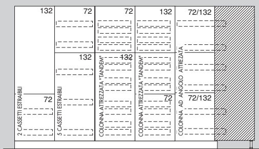
COLONNE ATTEZZATE EQUIPPED TALL UNITS ARMOIRES EQUIPES H 204cm
