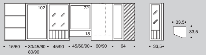
PENSILI WALL UNITS ÉLÉMENTS HAUTS H 102/132cm
