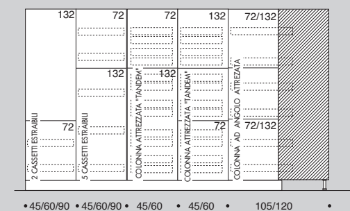
COLONNE ATTEZZATE EQUIPPED TALL UNITS ARMOIRES EQUIPES H 204cm
