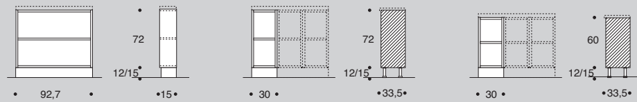
BASI A GIORNO OPEN BASE ÉLÉMENTS BAS OUVERTS
