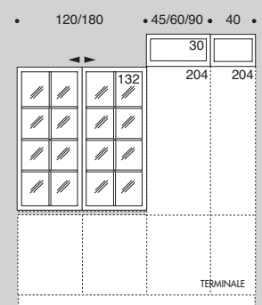
SOPRAPENSILE E SOPRACOLONNE SUSPENDED WALL UNIT AND TALL UNITS ELEMENTS SUR MEUBLES HAUTS ET SUR ARMOIRES
