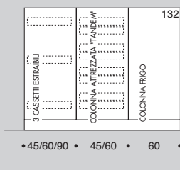
COLONNE ATTEZZATE EQUIPPED TALL UNITS ARMOIRES EQUIPES H 132cm
