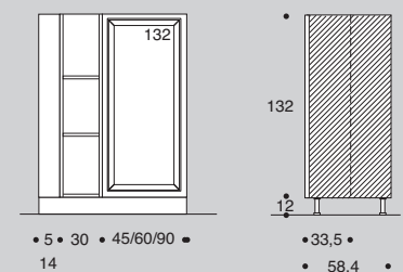
COLONNE TALL UNITS ARMOIRES H 132cm
