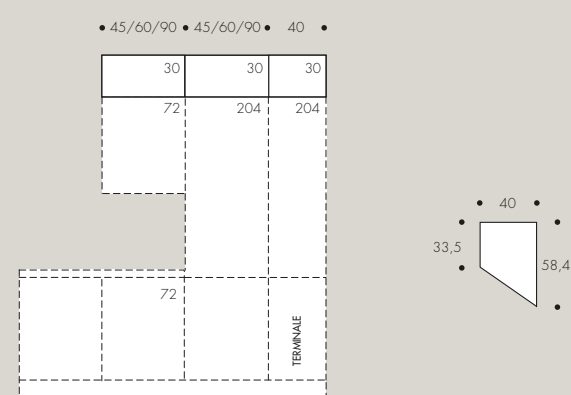
SOPRAPENSILE E SOPRACOLONNE SUSPENDED WALL UNIT AND TALL UNITS ELEMENTS SUR MEUBLES HAUTS ET SUR ARMOIRES
